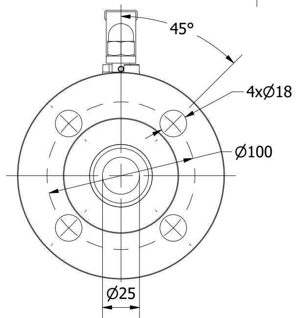
VIEW A-A
