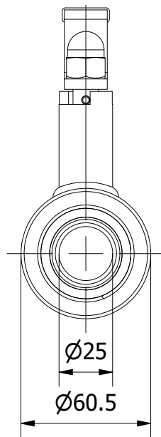
VIEW A-A
