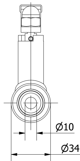
VIEW A-A
