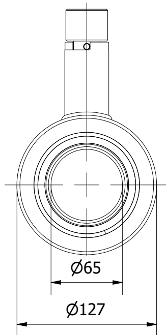
VIEW A-A
