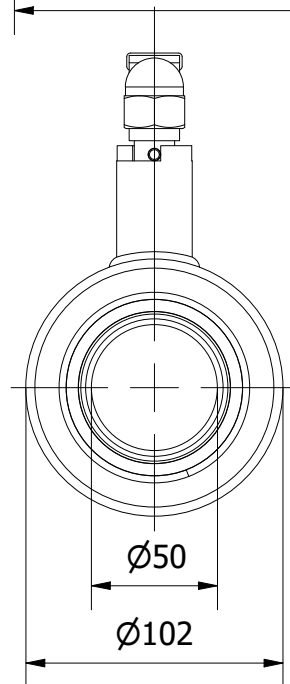
VIEW A-A
