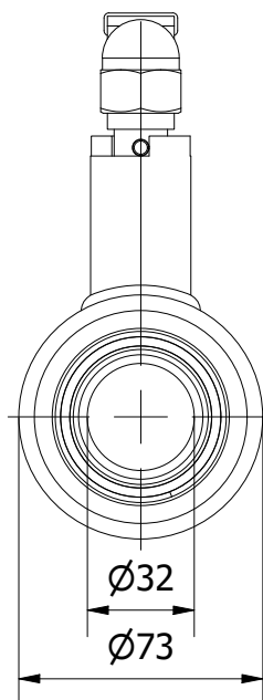
VIEW A-A
