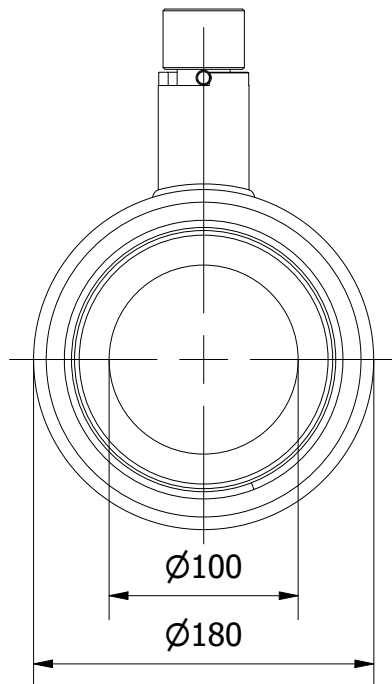
VIEW A-A
