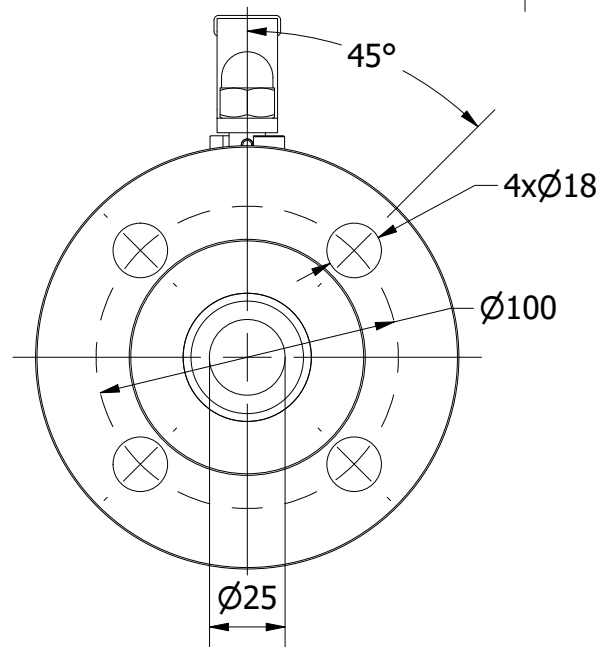
VIEW A-A
