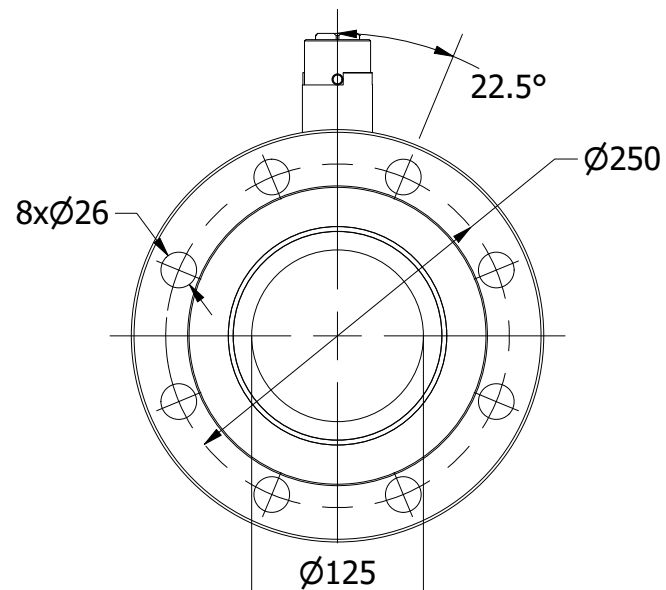
VIEW A-A
