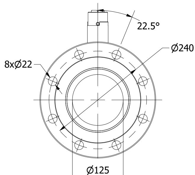
VIEW A-A
