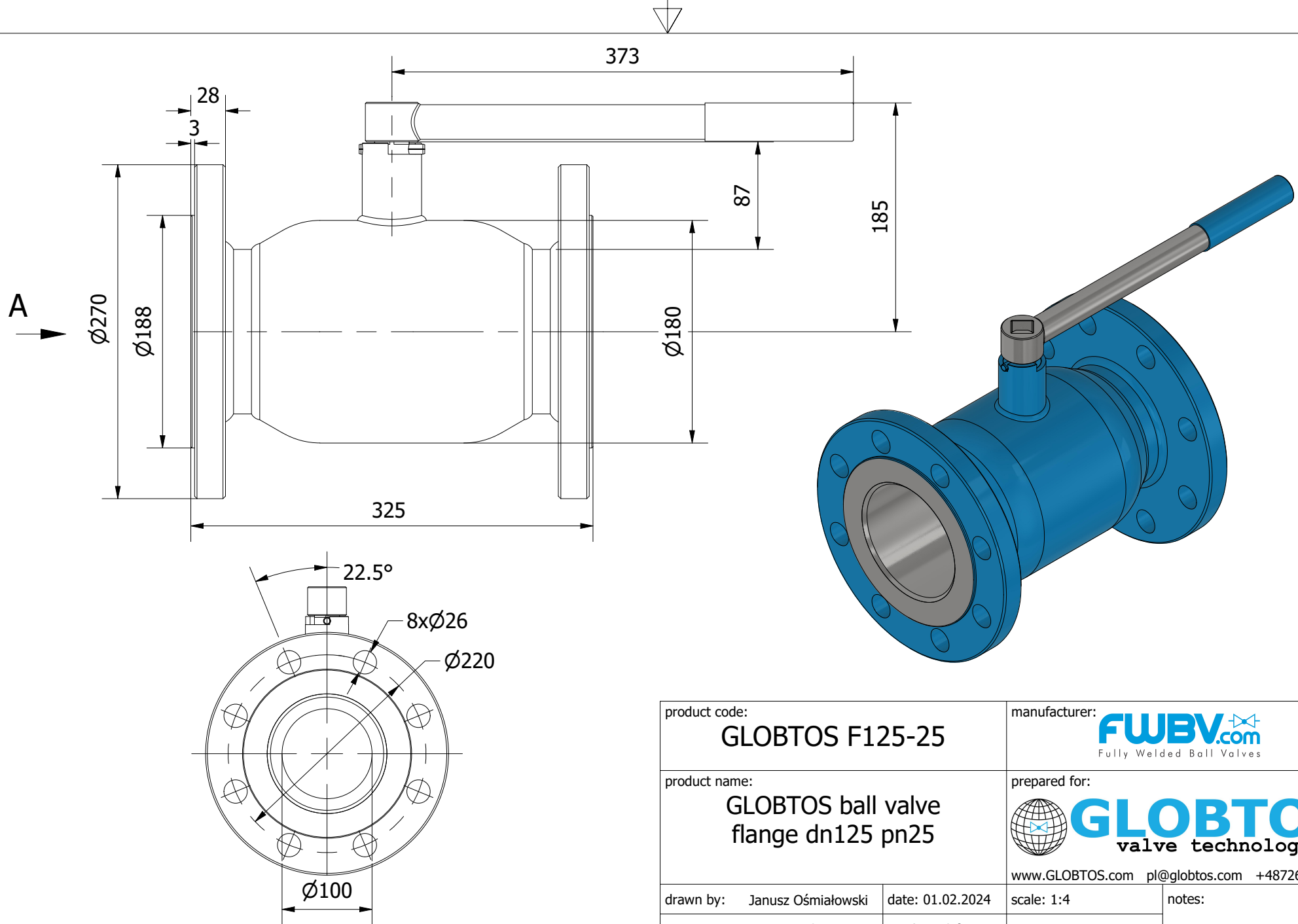
VIEW A-A
