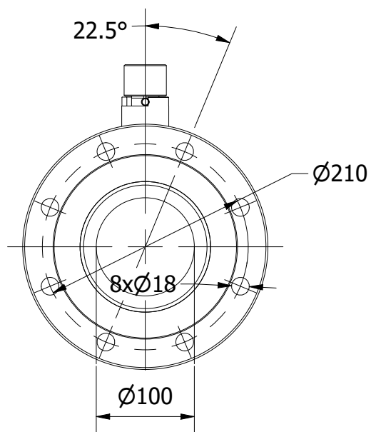
VIEW A-A
