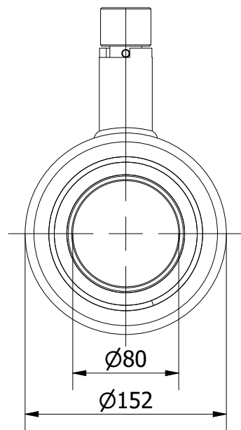
VIEW A-A
