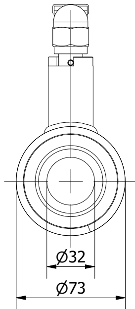
VIEW A-A
