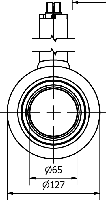
VIEW A-A
