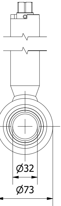
VIEW A-A
