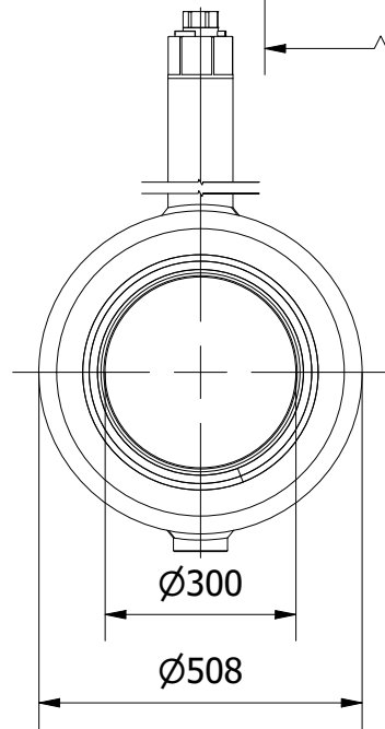
VIEW A-A
