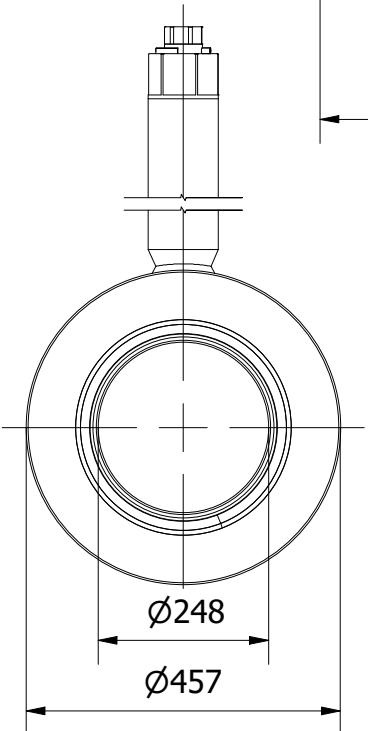
VIEW A-A
