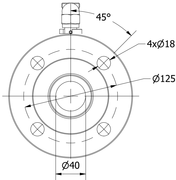
VIEW A-A
