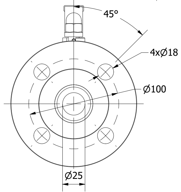
VIEW A-A
