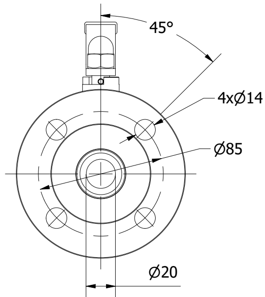
VIEW A-A
